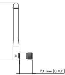
Antenna
