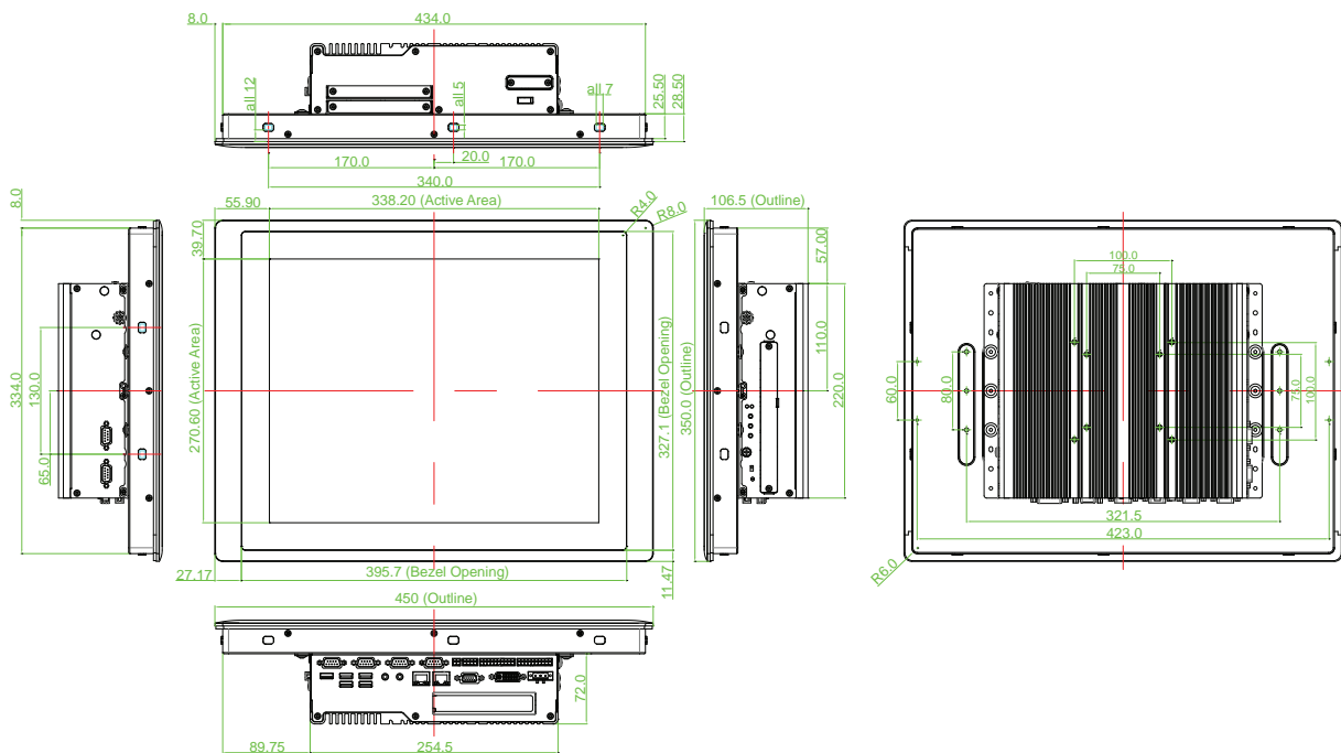
CV-117/P2002E
