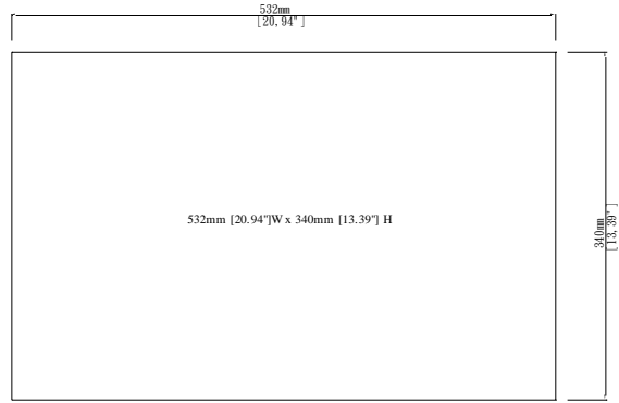
Cutout Dimensions
